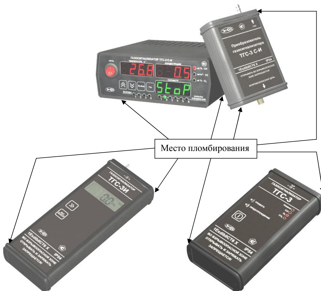
Рисунок 4 – Схема пломбирования корпуса газосигнализатора ТГС-3
